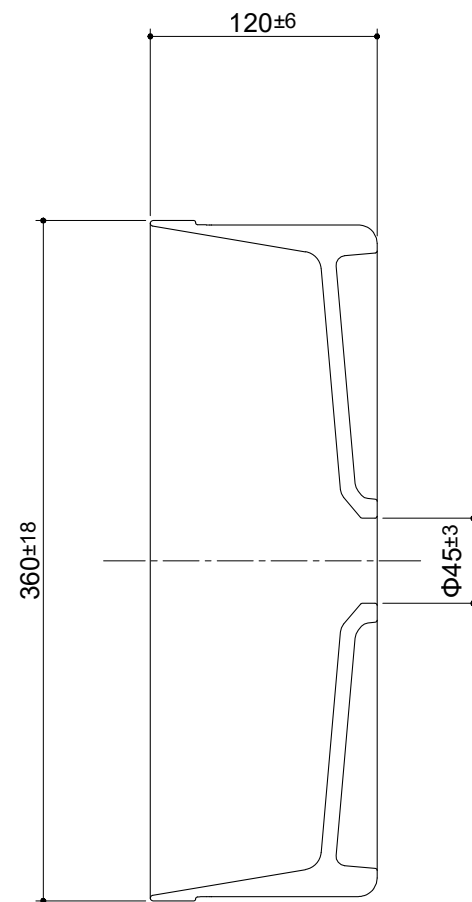
Section A-A
