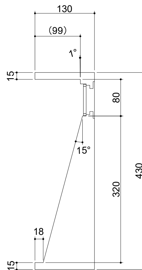
Section A-A
